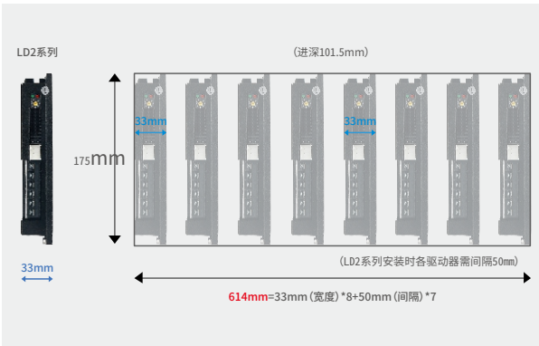
单轴
