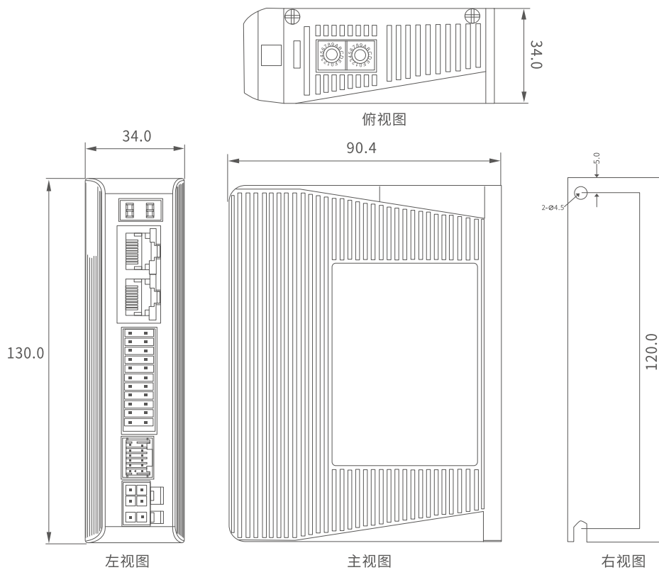
CL3-EC503/CL3-EC507驱动器尺寸图 (单位mm)
