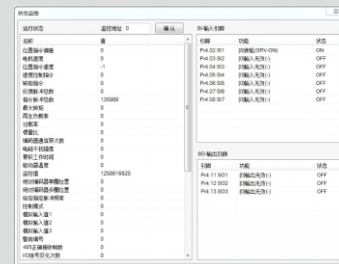
状态监控： 输入输出接口实时状态监控
