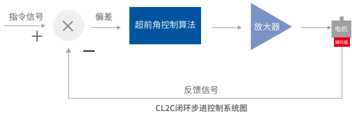
CL2C闭环步进控制系统图
