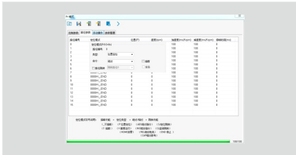
路径参数 16段路径程序编写。进行位置、速度、回原点等多种运动控制程序的具体参数设置
