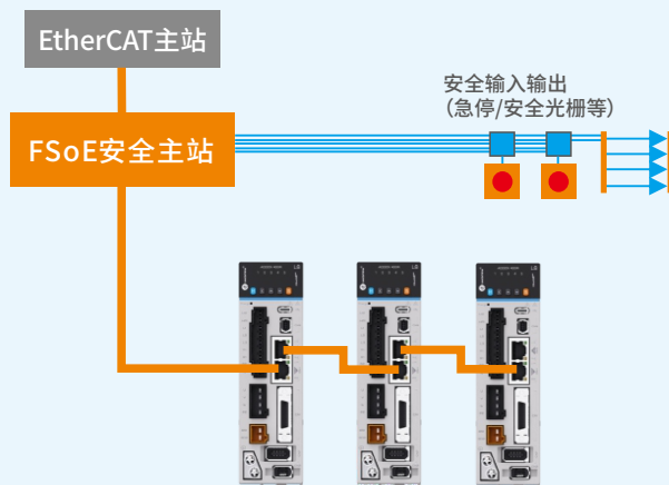
FSoE总线功能安全方案系统拓扑图
