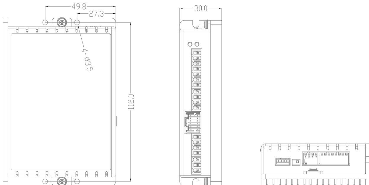
CL1-728安装尺寸图 单位 (mm)
