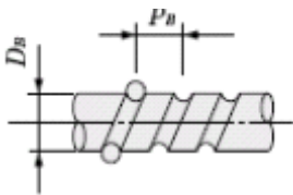
图2：丝杠参数
