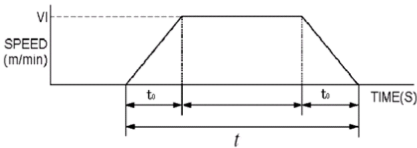
图3：运行曲线
