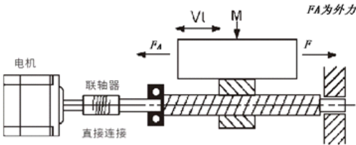
图1：丝杠水平运动
