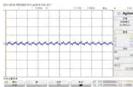
图7 57CM23电机在900rpm时的绕组电流波形
