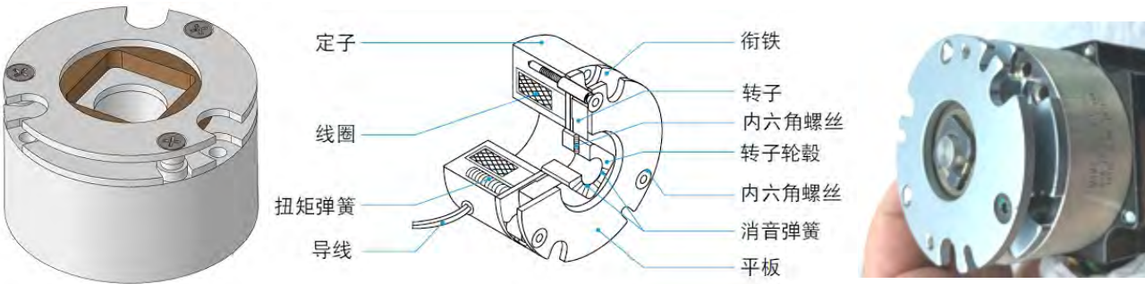
结构3D图
