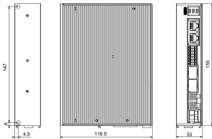
2DM3-EC882S安装尺寸图
