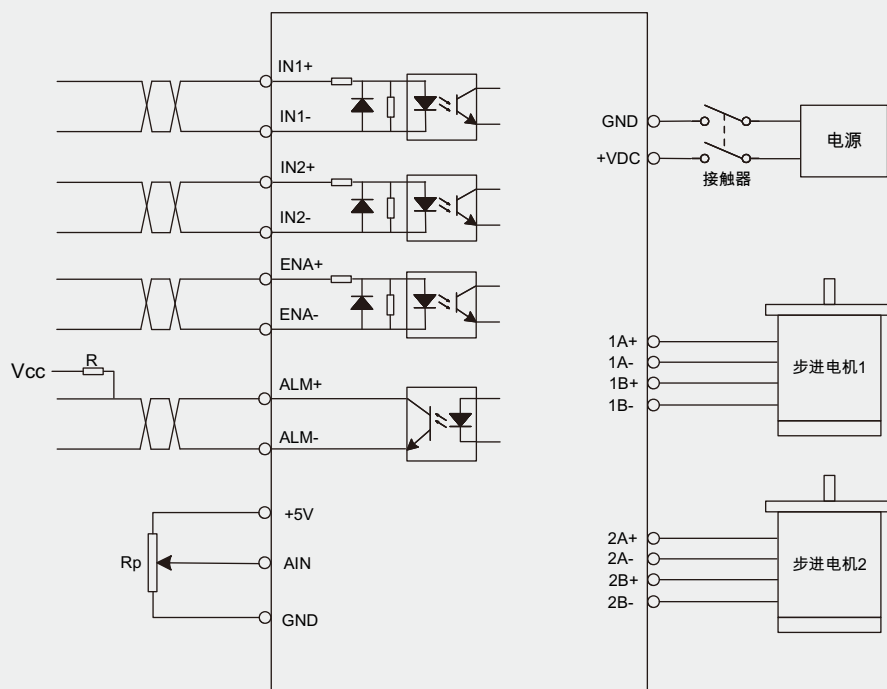
2DM57C-A、2DM86C-A电气接线图
