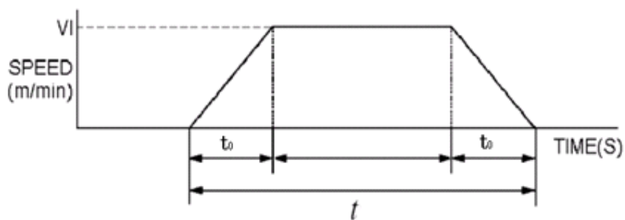
图3：运行曲线
