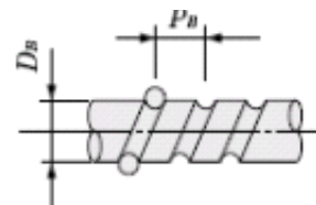
图2：丝杠参数
