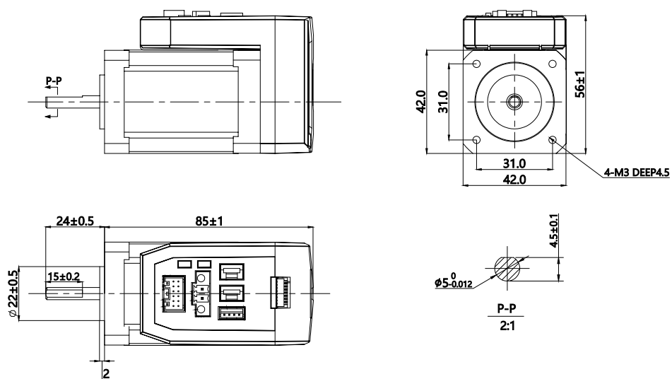
iDM42-RS08 (V2.0)
