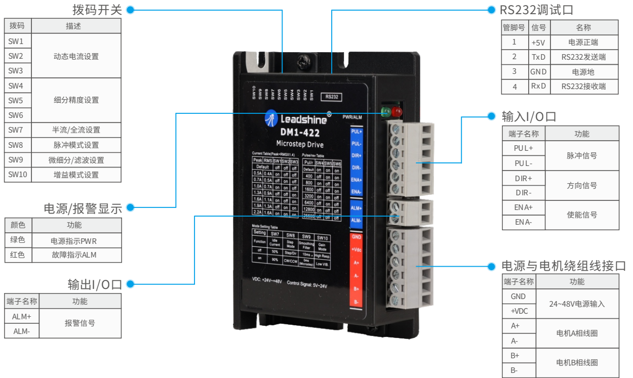
DM1-422、DM1-432接口说明
