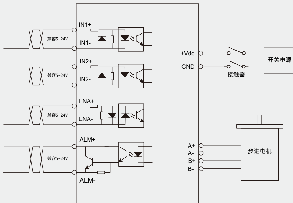
DM1-IO422C、DM1-IO442C、DM1-IO542C、DM1-IO556C电气接线图
