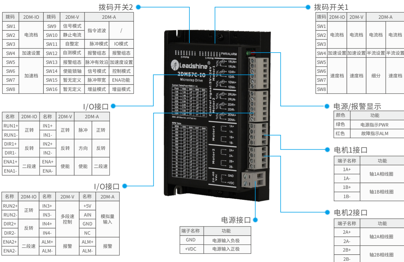
2DM57C-IO/-V/-A接口示意图
