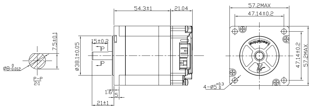
iCL57A-RS13
