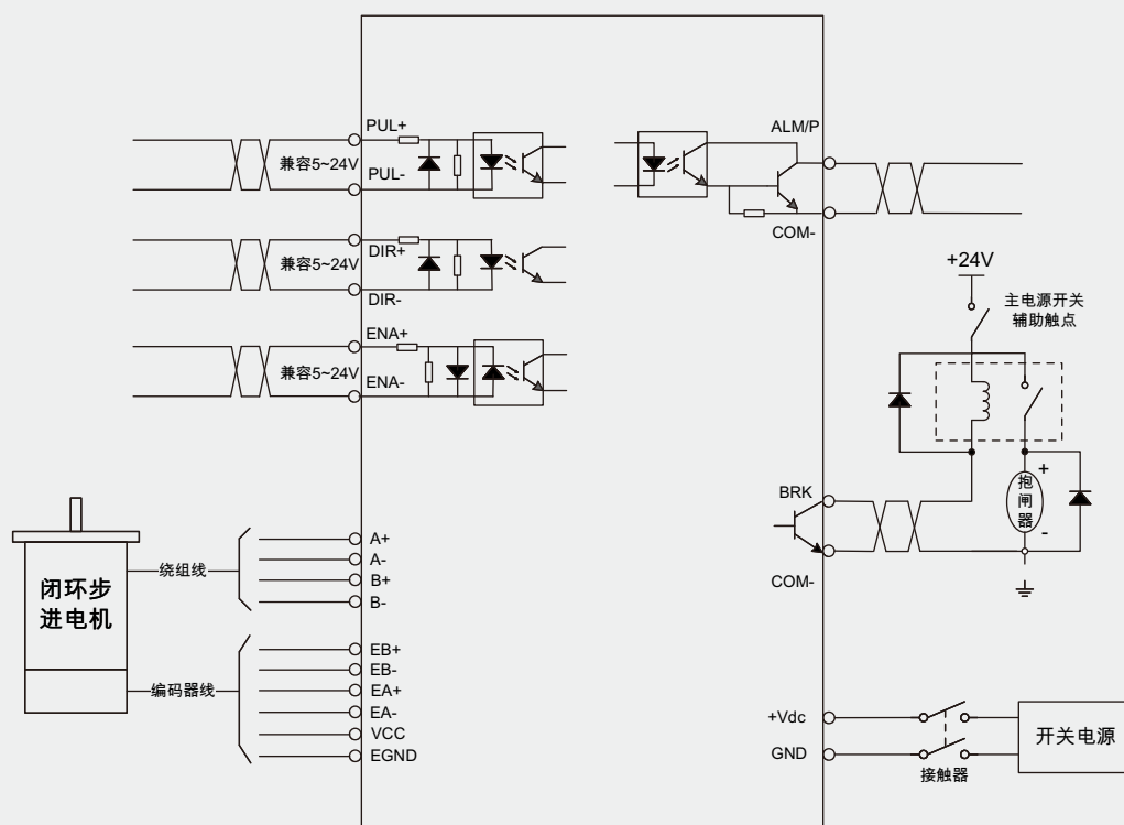
CL1-42C/57C电气接线图
