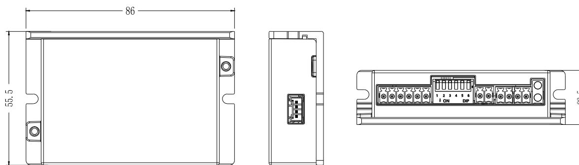
DM1-422C、DM1-432C安装尺寸图
