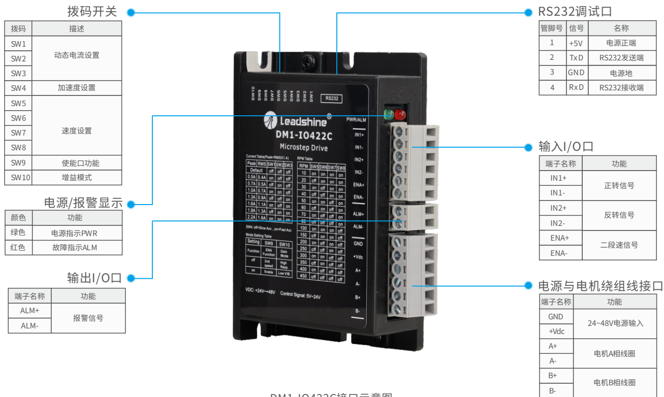
DM1-IO422C接口示意图
