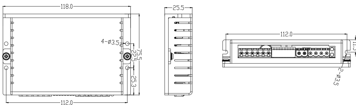
DM1-542C、DM1-556C安装尺寸图
