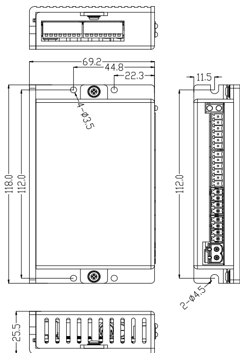
2DM42T 安装尺寸图
