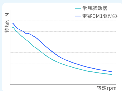
DM1系列驱动器与传统驱动器匹配统一电机(同一条件)的转矩图
