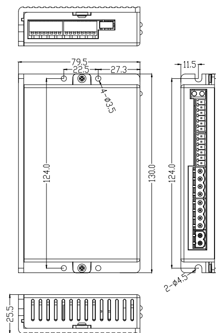
2DM86C-IO/-V/-A安装尺寸图
