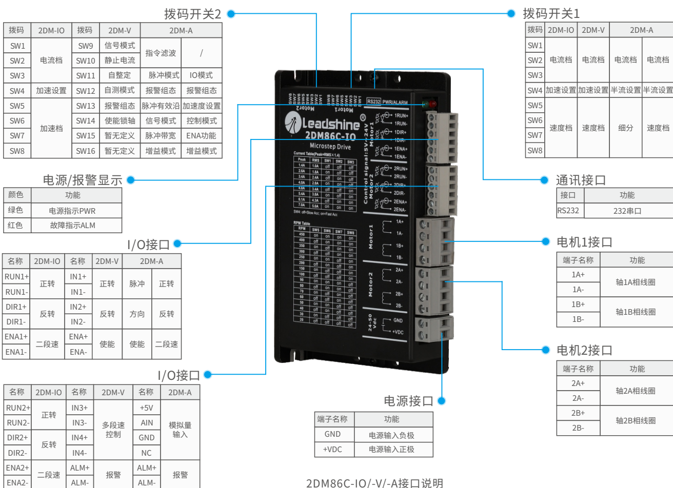
2DM86C-IO/-V/-A接口说明
