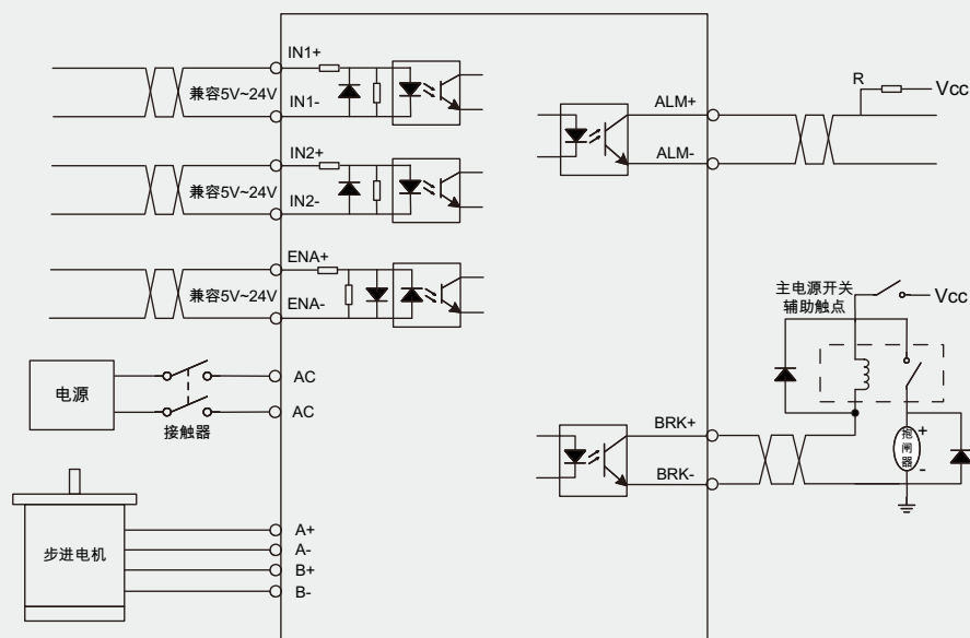
DM1-IO860C电气接线图
