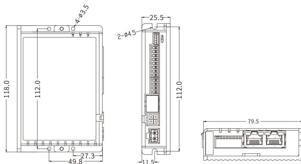
DM2B-RS522/542/556/570安装尺寸图
