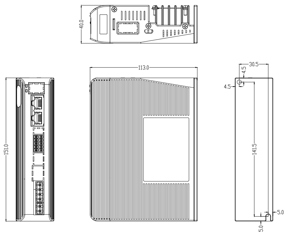
DM3B-EC882AC安装尺寸图
