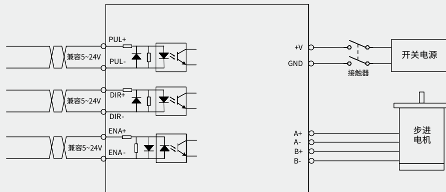
DM1-422C、DM1-432C、DM1-442C、DM1-542C、DM1-556C接线图
