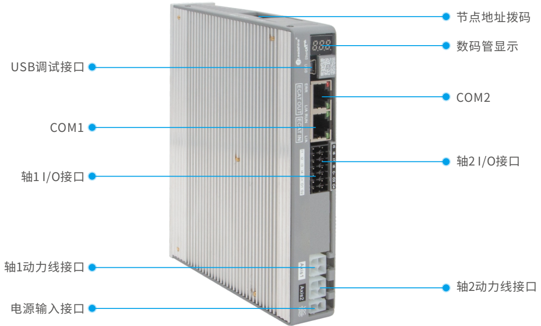
2DM3-EIP522/556/870接口说明
