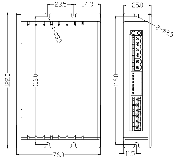
DM1-IO442C安装尺寸图
