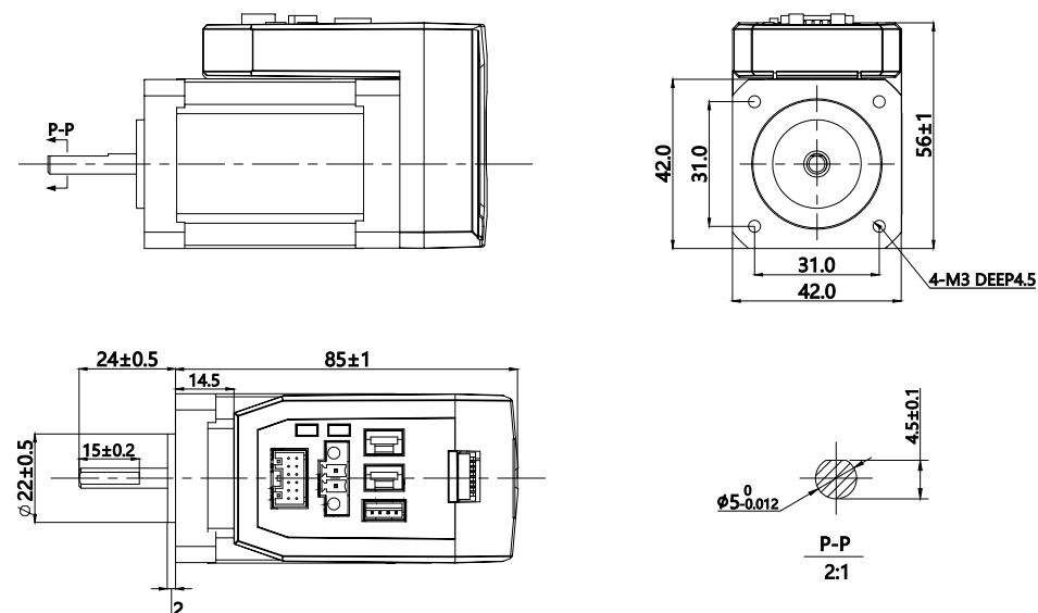
iCL42-RS08 (V2.0)
