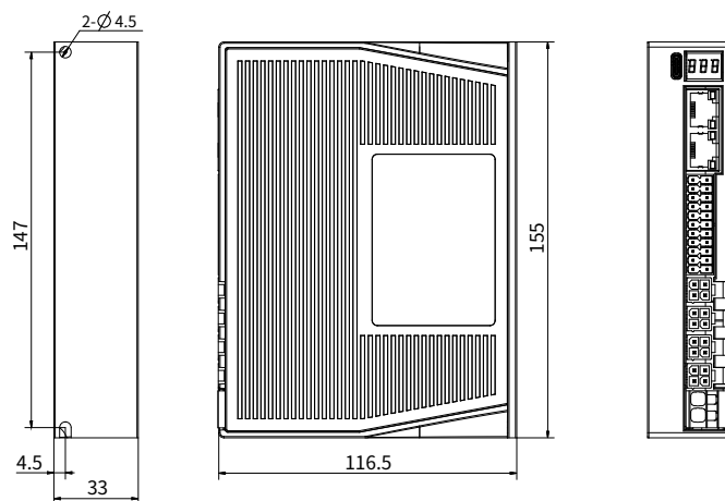
4DM3C-EC432/556 安装尺寸图
