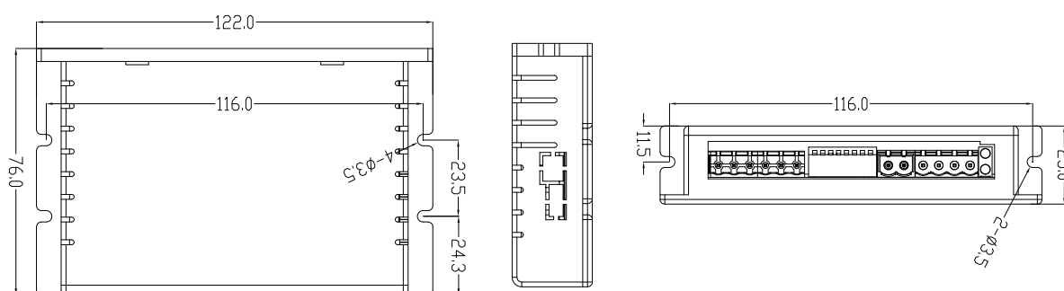
DM1-442C安装尺寸图
