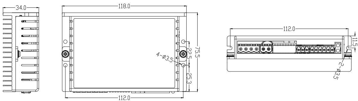
DM1-556、DM1-870安装尺寸图
