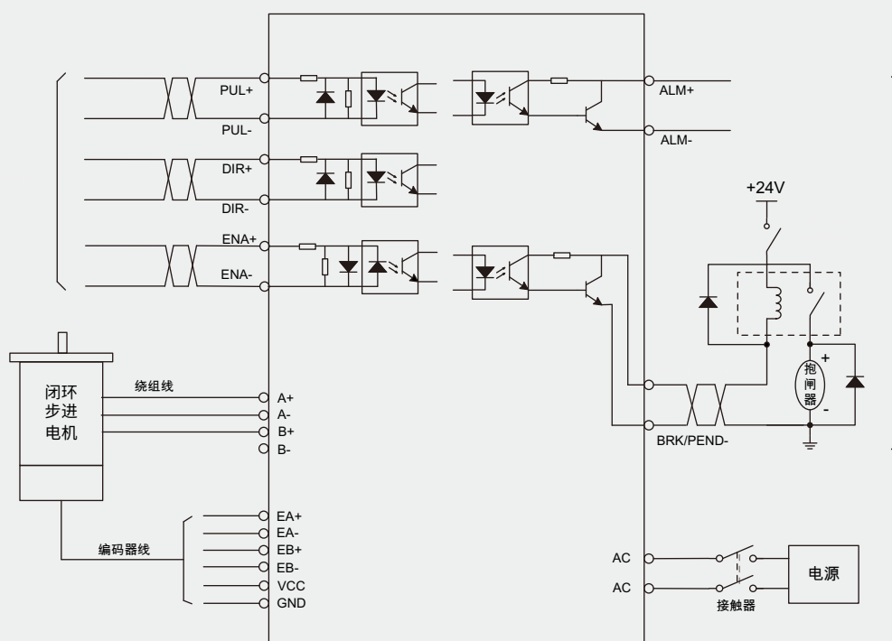
CL1-86C电气接线图
