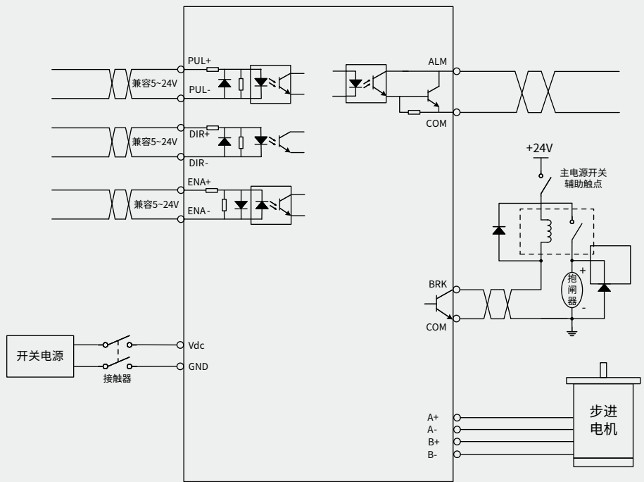
DM1-542、DM1-556、DM1-870接线图
