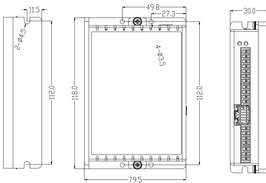
CL1-728安装尺寸图
