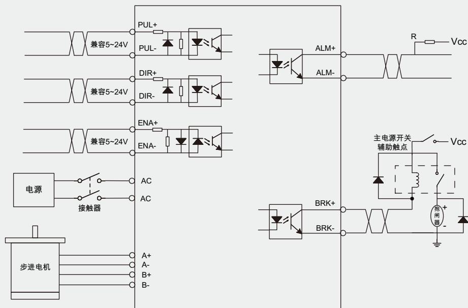
DM1-860C接线图
