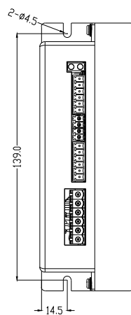
CL1-86C安装尺寸图
