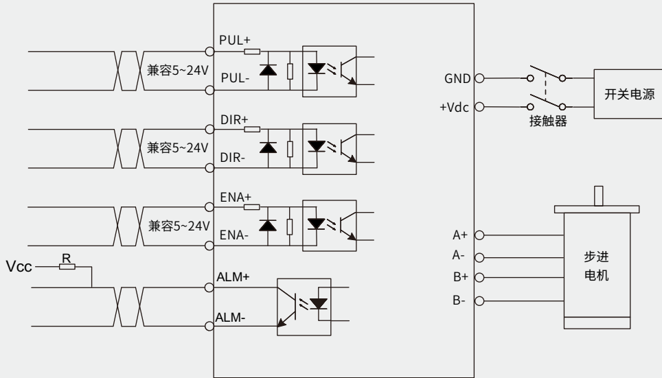
DM1-422、DM1-432接线图
