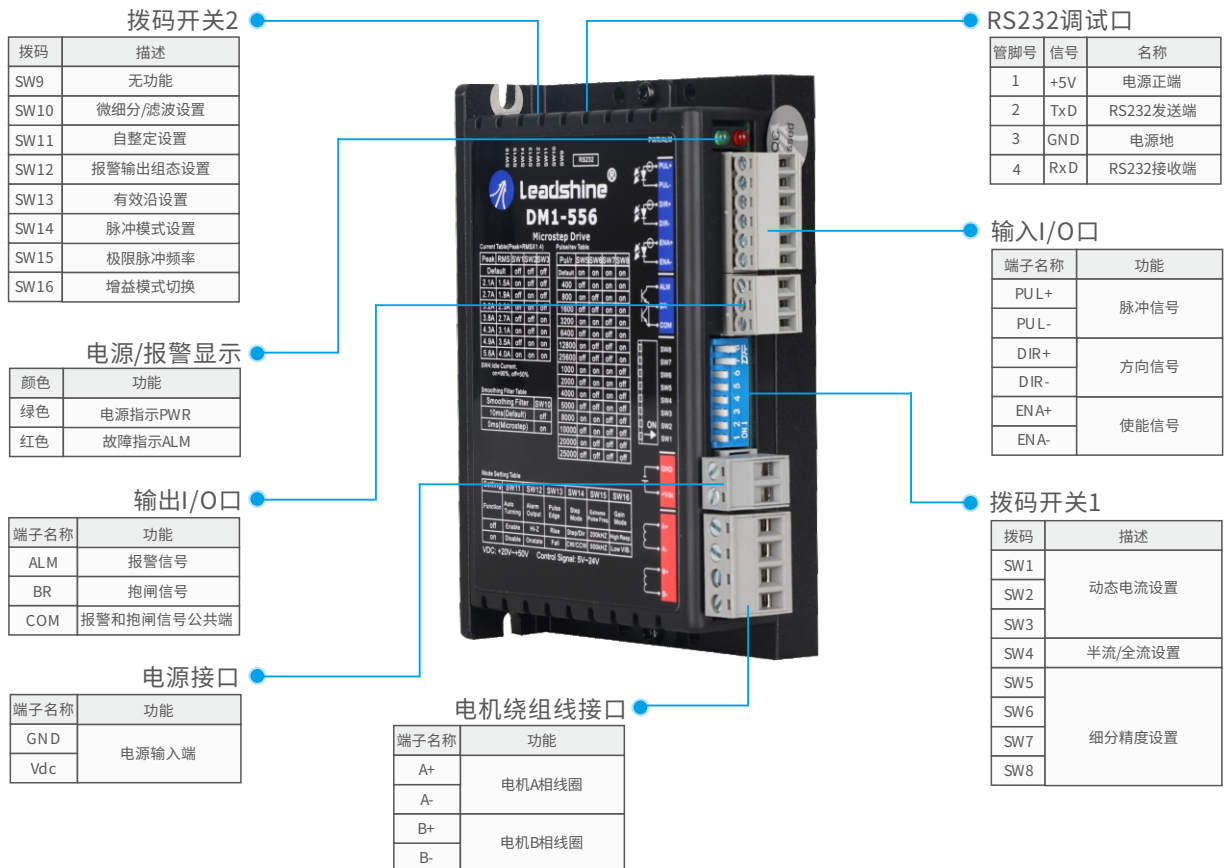
DM1-542、DM1-556、DM1-870接口说明
