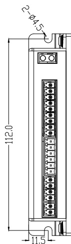
CL1-42C/57C安装尺寸图
