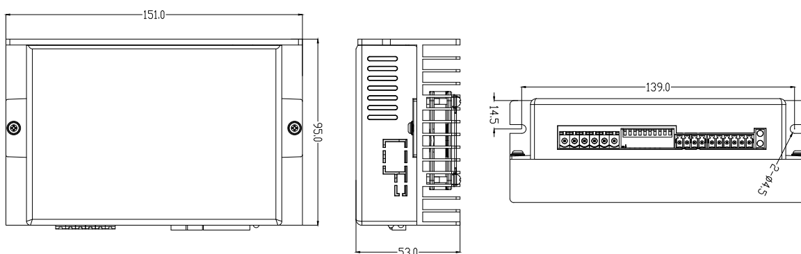
DM1-860C安装尺寸图
