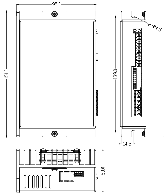
DM1-IO860C安装尺寸图
