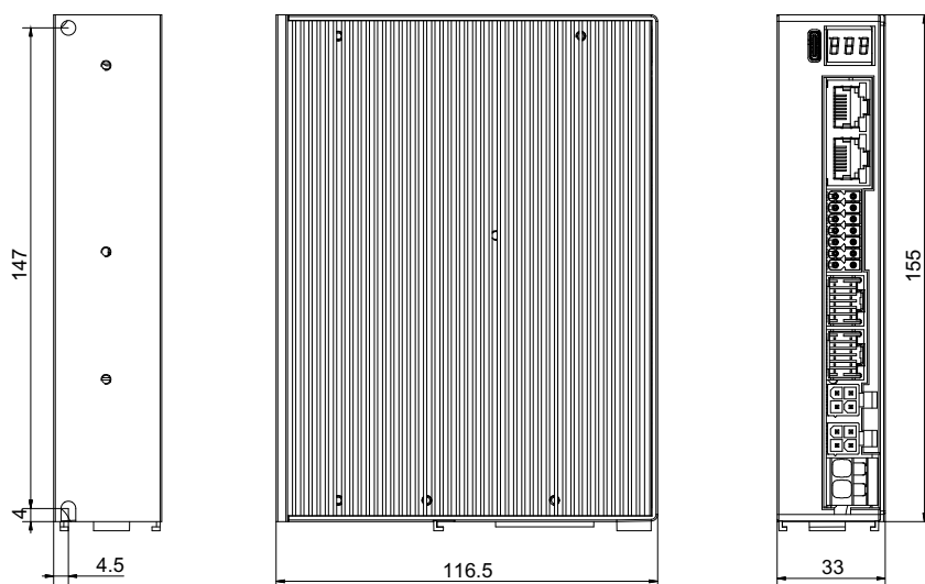
2CL3-EC808T安装尺寸图
